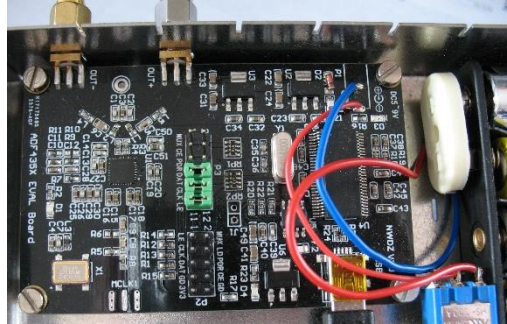
ADF4351 Ref 25MHz
