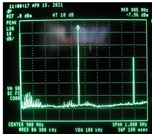
ADF4351 Ref 25MHz
