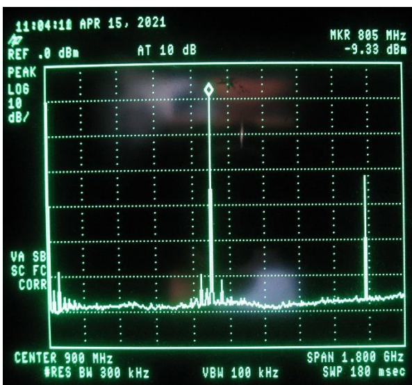
MAX2870 800MHz
