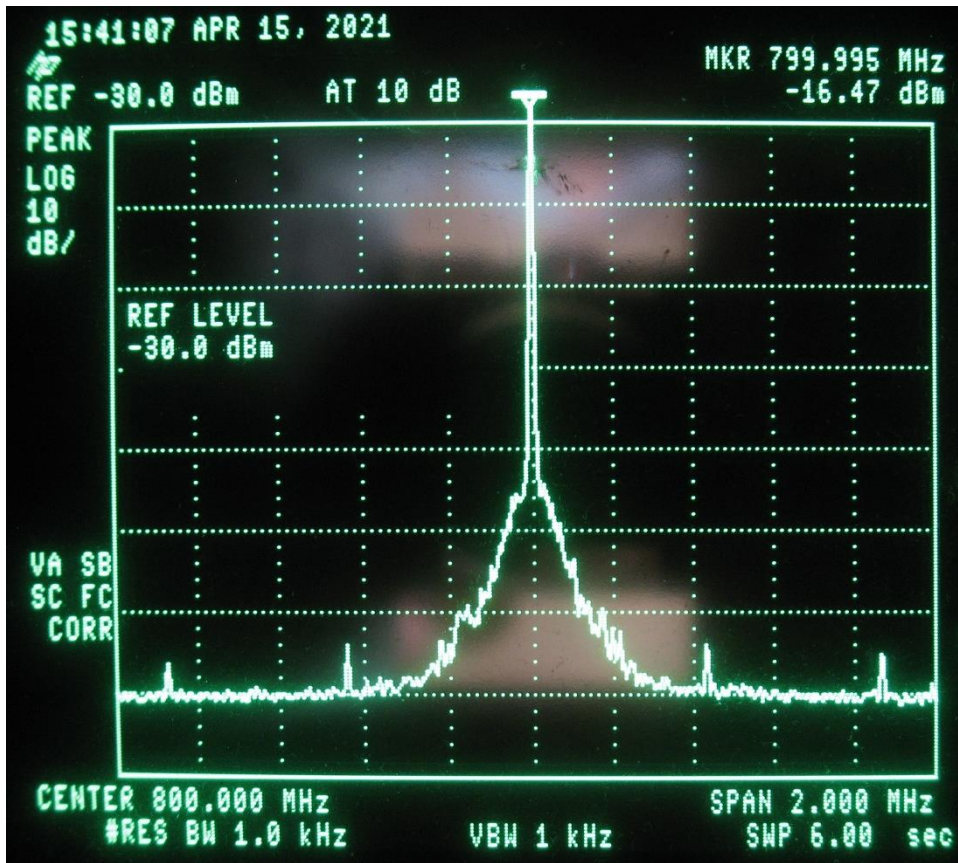
MAX2870 800MHz (Pegelmessung in Begrenzung)
