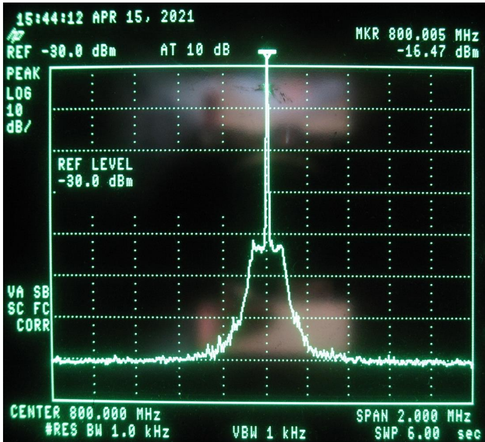
ADF4351 800MHz (Pegelmessung in Begrenzung)
