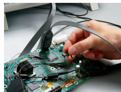
Der Digitalstastkopf P6316 für die MSO2000-Serie vereinfacht die Verbindung zum Prüfling
