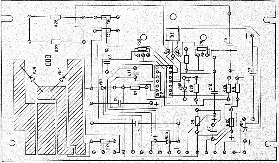
LEITERPLATTE 008
