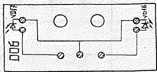
LEITERPLATTE 006
