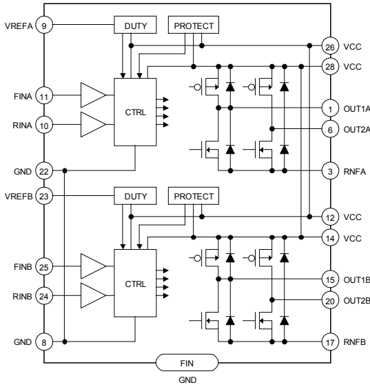
Fig.33 BD6236FM
