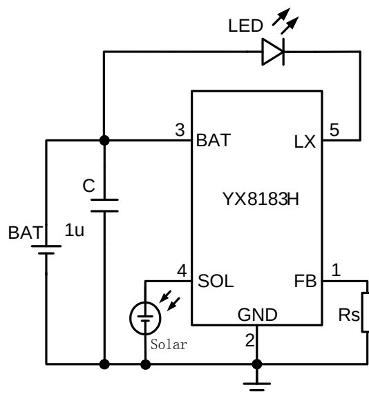
图 3 方案一：直驱方案
