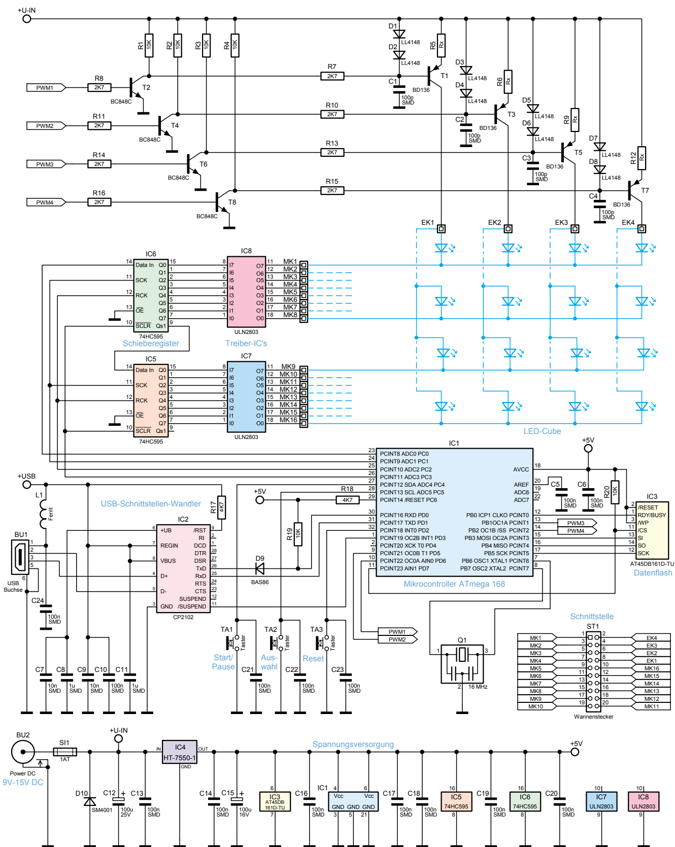
Bild 3: Die Gesamtschaltung des LED-Cubes
