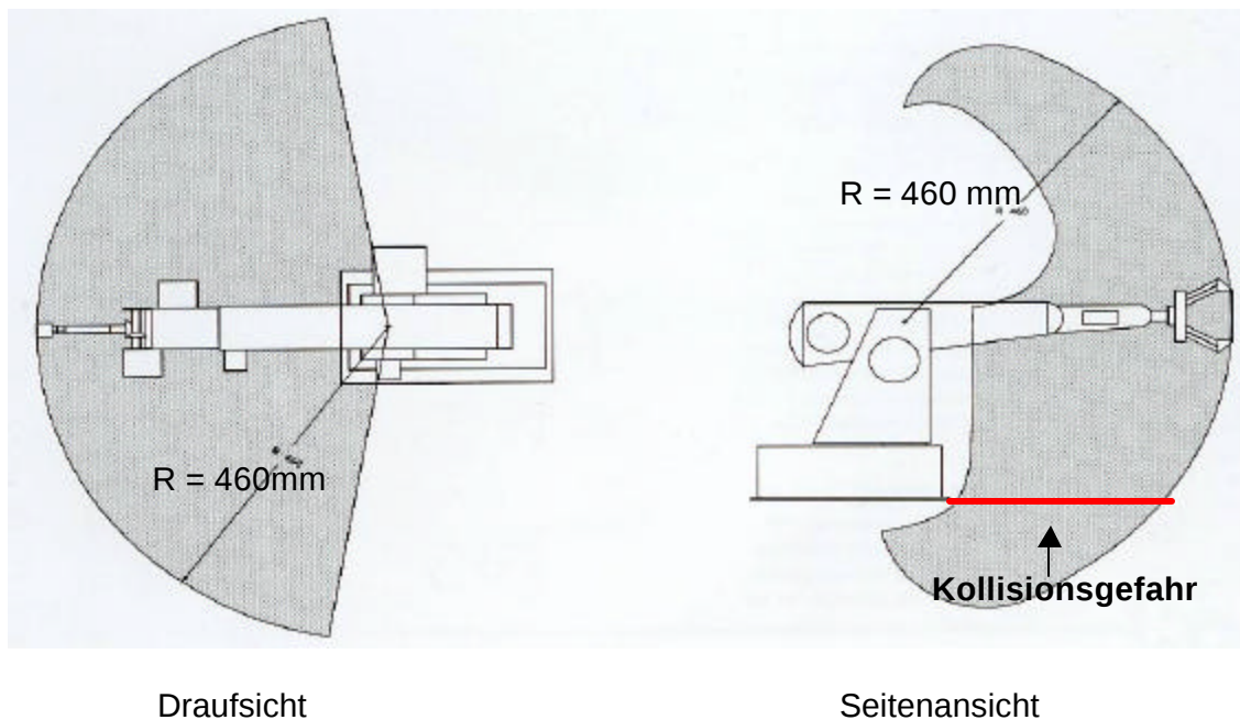
Abbildung 3.4 : Der Arbeitsraum des Roboters ROB3 [8]
