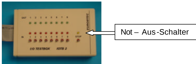
Abbildung 5.3 : Die I/O Testbox der Firma EUROBTEC
