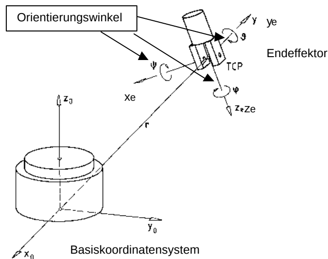
Abbildung 3.6 : Endeffektor mit Orientierungswinkel [5]
