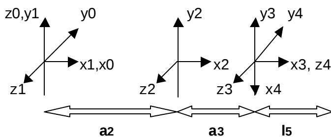
Abbildung 3.11 : Koordinatensystem der einzelnen Achsen
