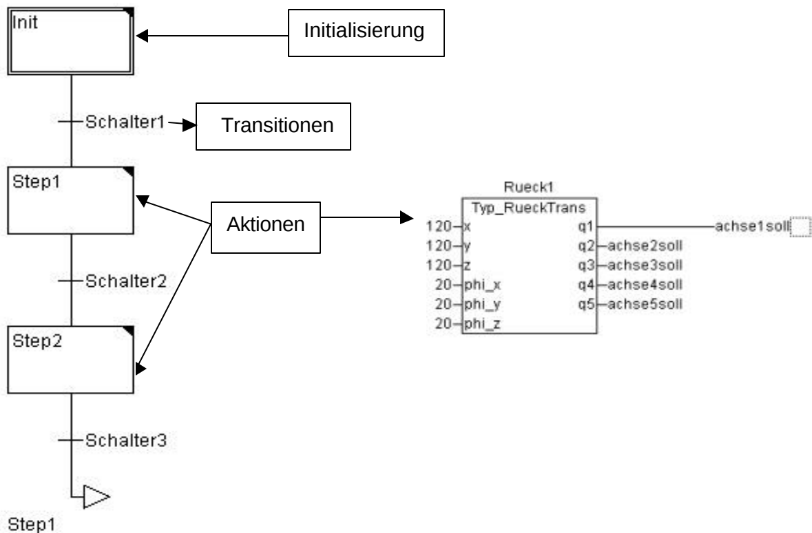
Abbildung 6.1 : Ablaufsprachen-Editor
