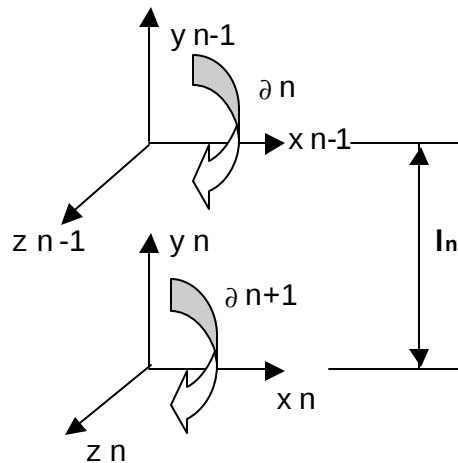
Abbildung 3.9 : Lotrechte Verschiebung zwischen zwei benachbarten Gelenken
