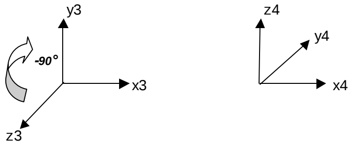
Abbildung 3.13 : Drehung um die x – Achse bei letztem Gelenk
