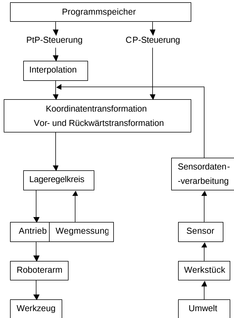
Abbildung 2.2 : Informationsfluss bei einer Robotersteuerung [1]
