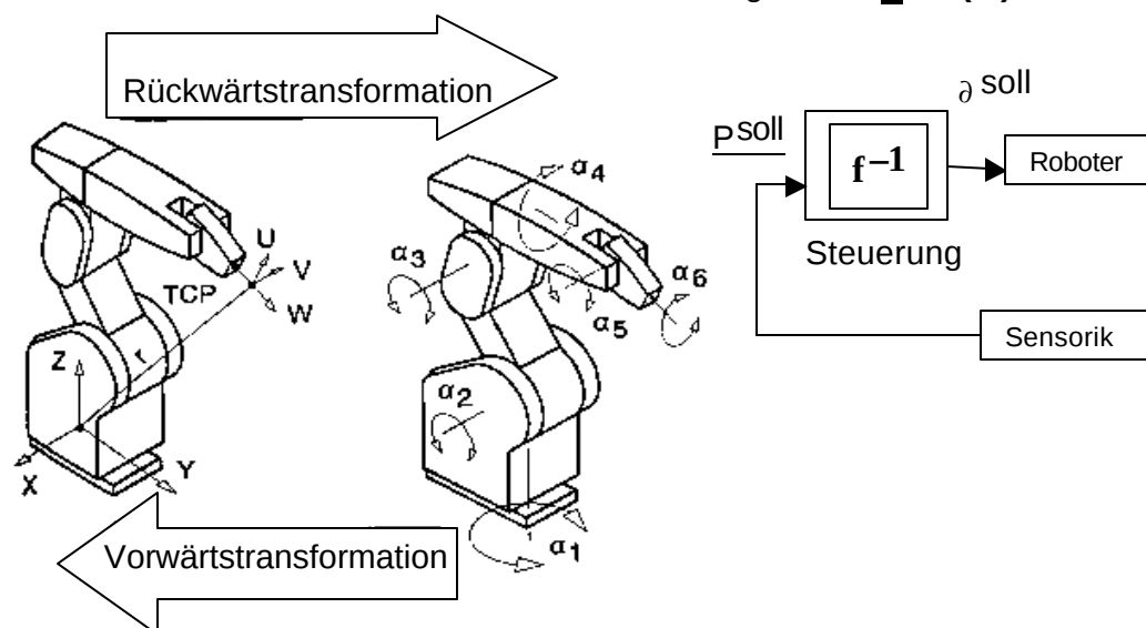
Abbildung 3.7 : Transformationen bei Robotersteuerung [1]
