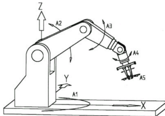
Abbildung 3.2 : Fünfgliedrige Trainingsroboter ROB 3
