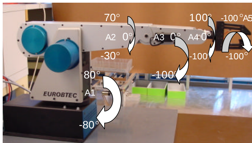
Abbildung 3.3 : Grundstellung des Trainingsroboters mit ROB 3
