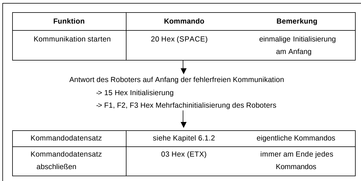
Abbildung 5.2 : Übersicht über den Kommunikationsablauf
