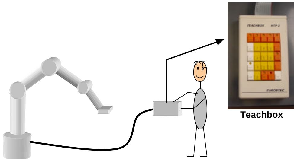
Abbildung 4.1 : Teach-in-Programmierung mit Teachbox des ROB 3
