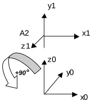
Abbildung 3.12 : Drehung um die x - Achse bei erstem Gelenk
