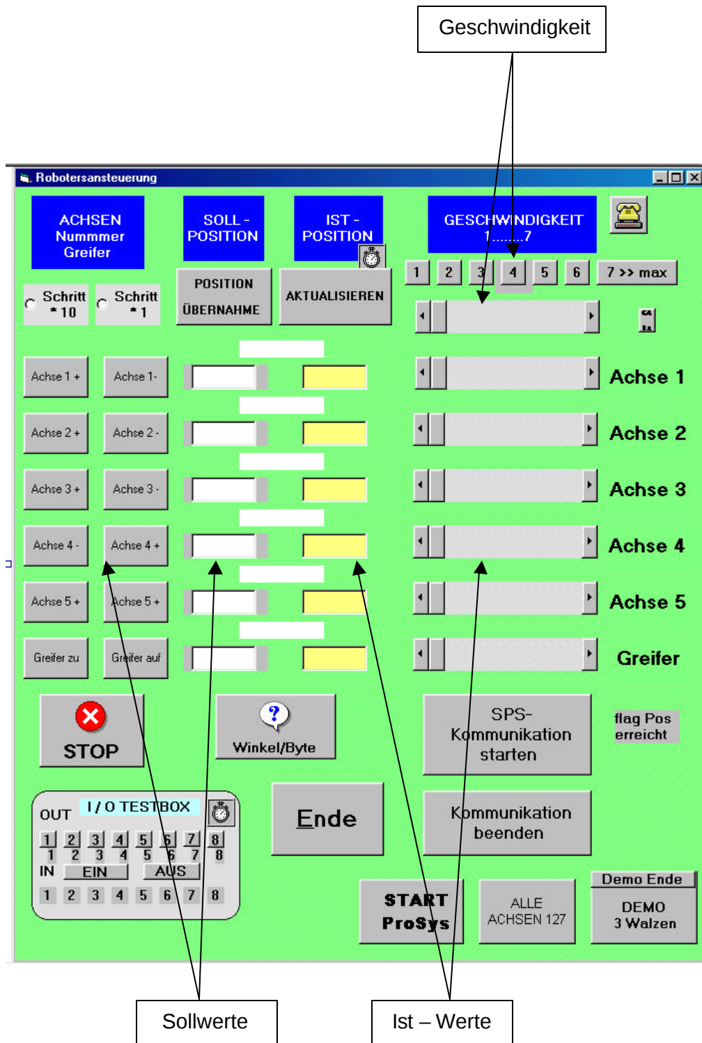
Abbildung 8.5 Hauptformular
