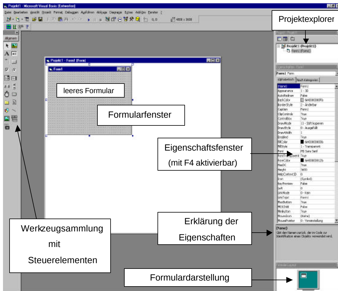
Abbildung 7.1 Visual - Basic - Entwicklungsumgebung
