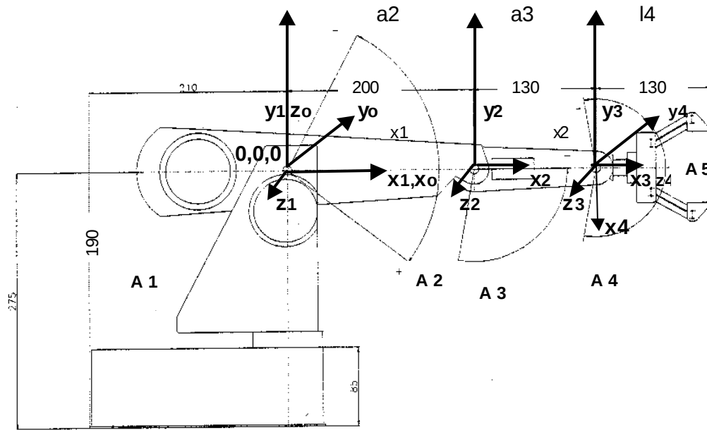
Abbildung 3.5 : Grundstellung des Roboterarmes mit Weltkoordinaten [7]
