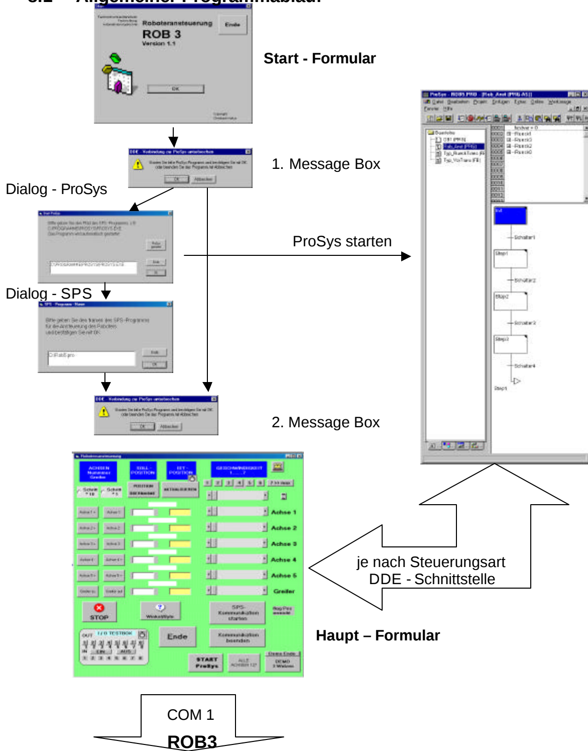
Abbildung 8.1 Programmablauf in der Ansteuerung des ROB3
