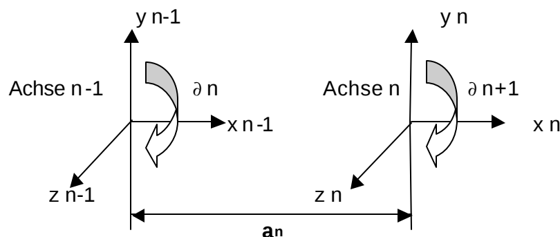
Abbildung 3.8 : Senkrechte Verschiebung zwischen benachbarten Gelenken
