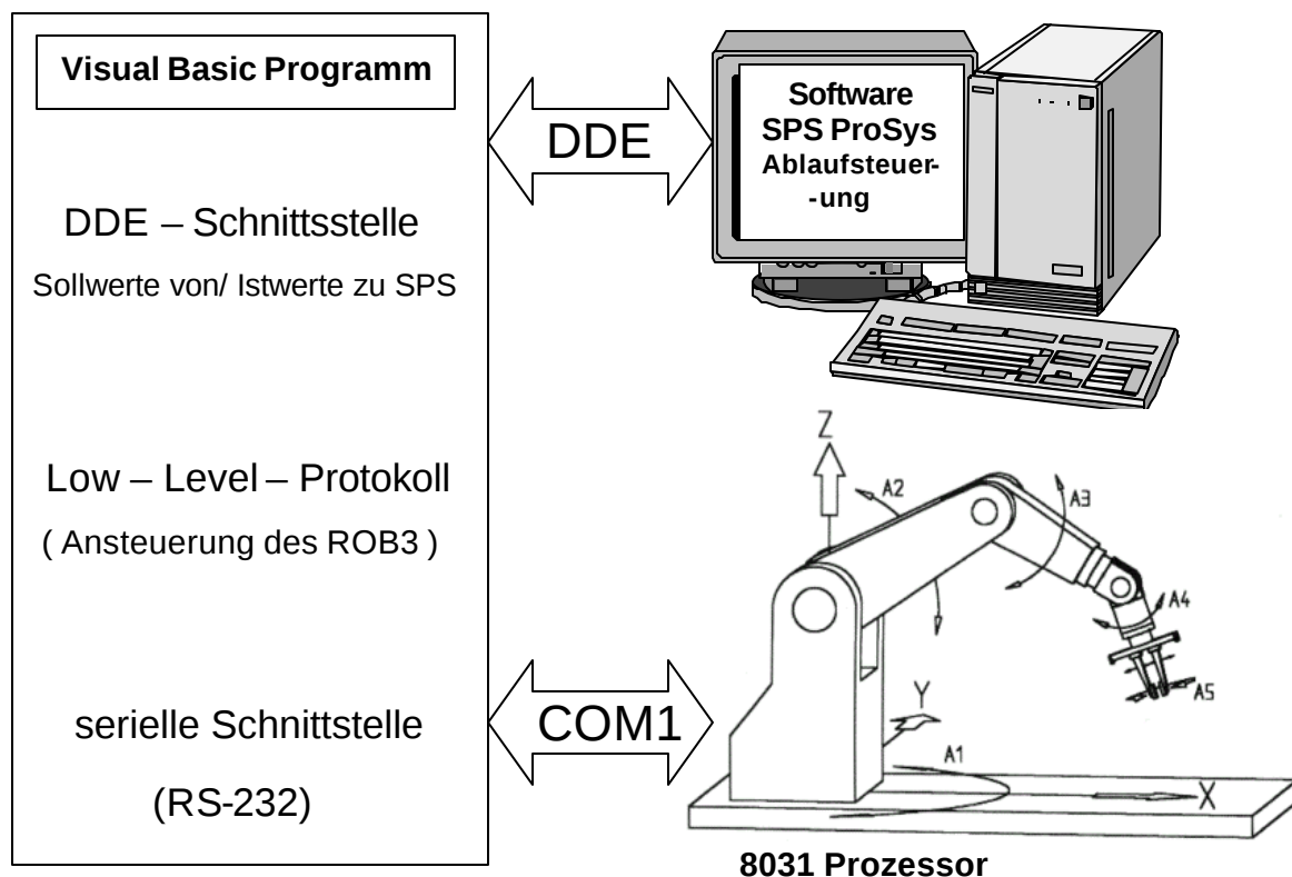
Abbildung 5.1. Prinzip der Programmierung und Ansteuerung des ROB3
