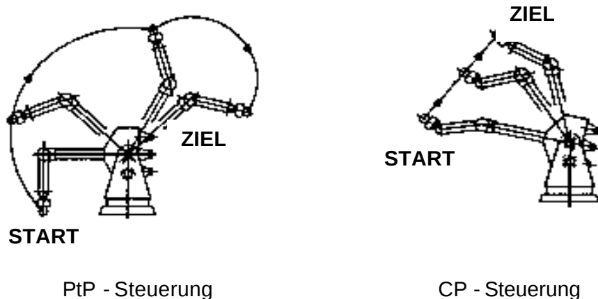
Abbildung 2.1 : Bewegungsarten eines Roboters[1]
