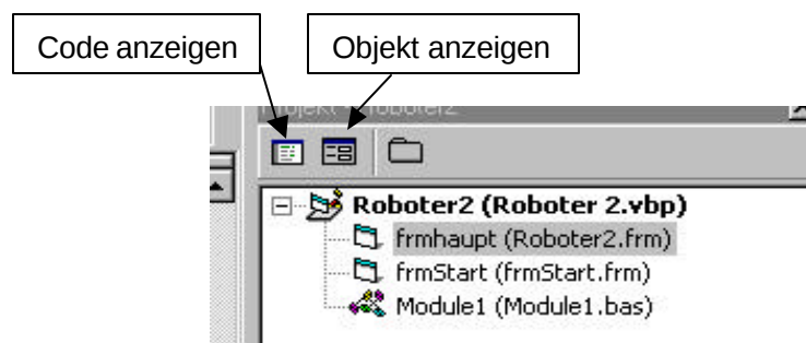
Abbildung 7.2 Projekt Explorer
