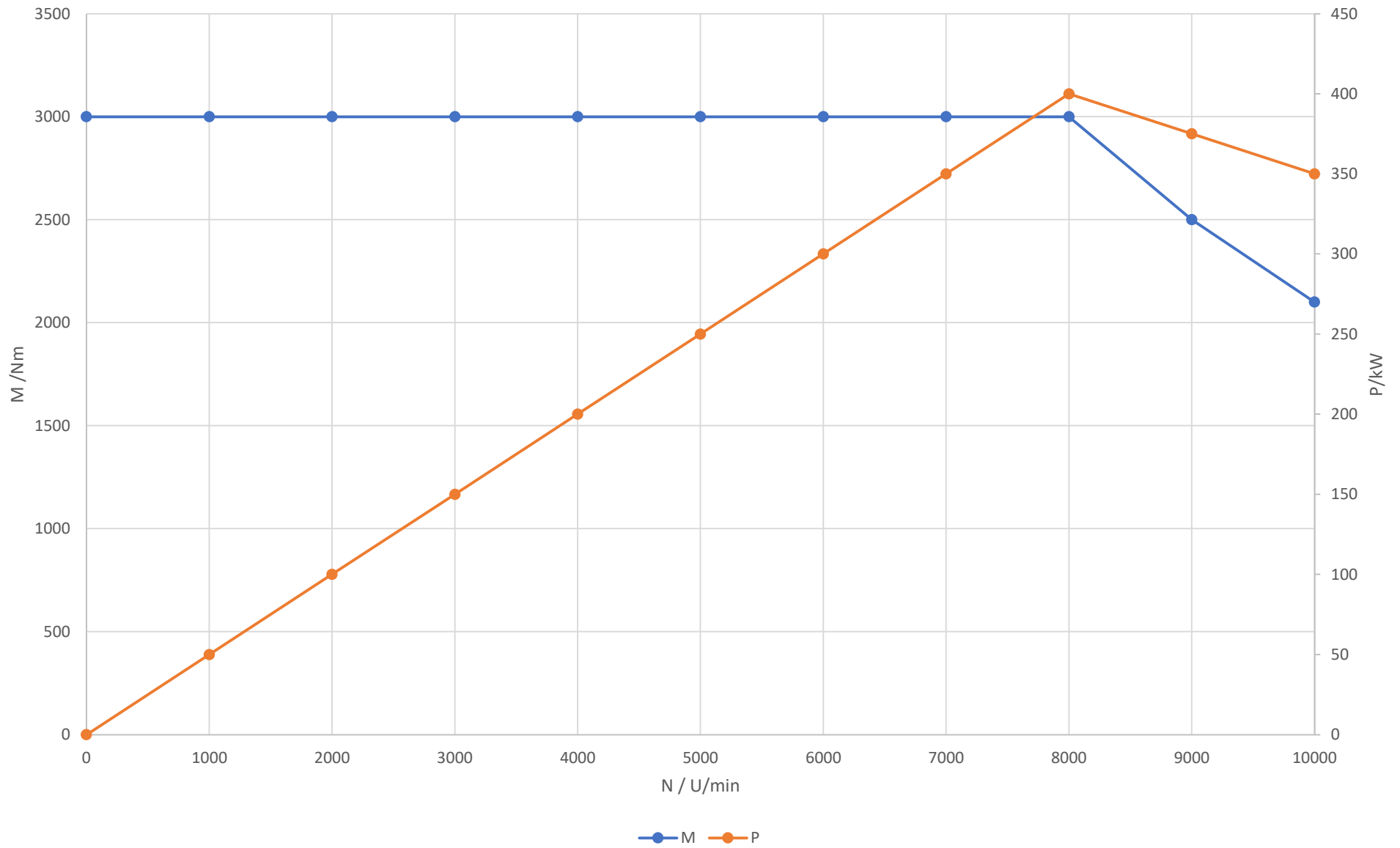
Motorkennlinie
