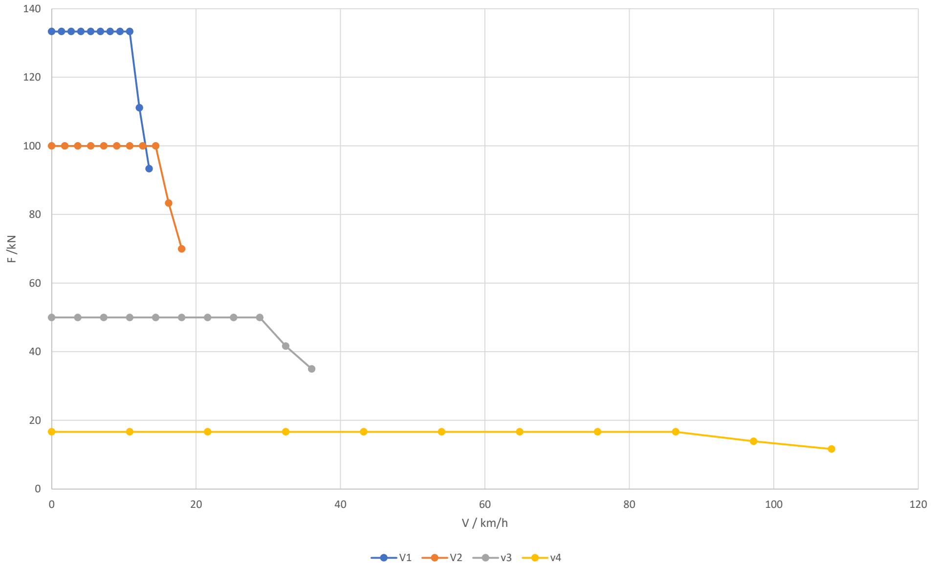
Kennlinie der Gänge
