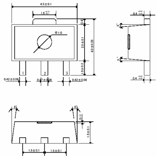
SOT-89
