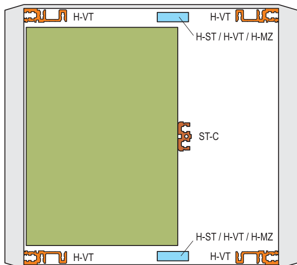
Gehäuse 6 HE
