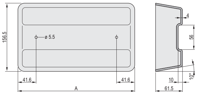
Kabelhalter
