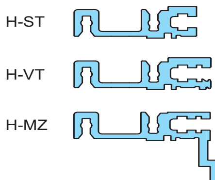
Modulschienen
