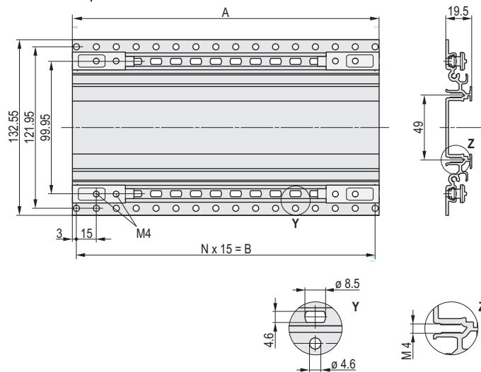
Seitenwandprofil 6 HE
