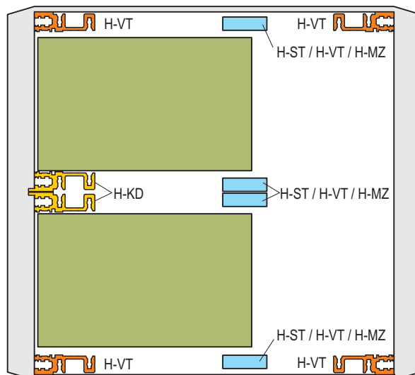
Modulschienen
