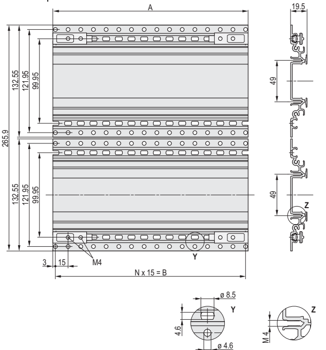
Seitenwandprofil 6 HE
