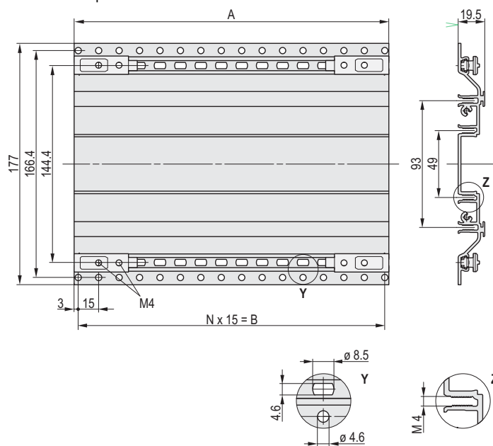
Seitenwandprofil 4 HE
