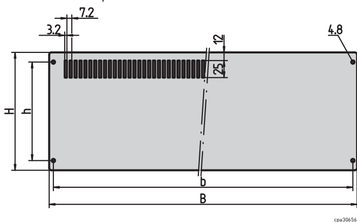
Rückwand / Frontplatte
