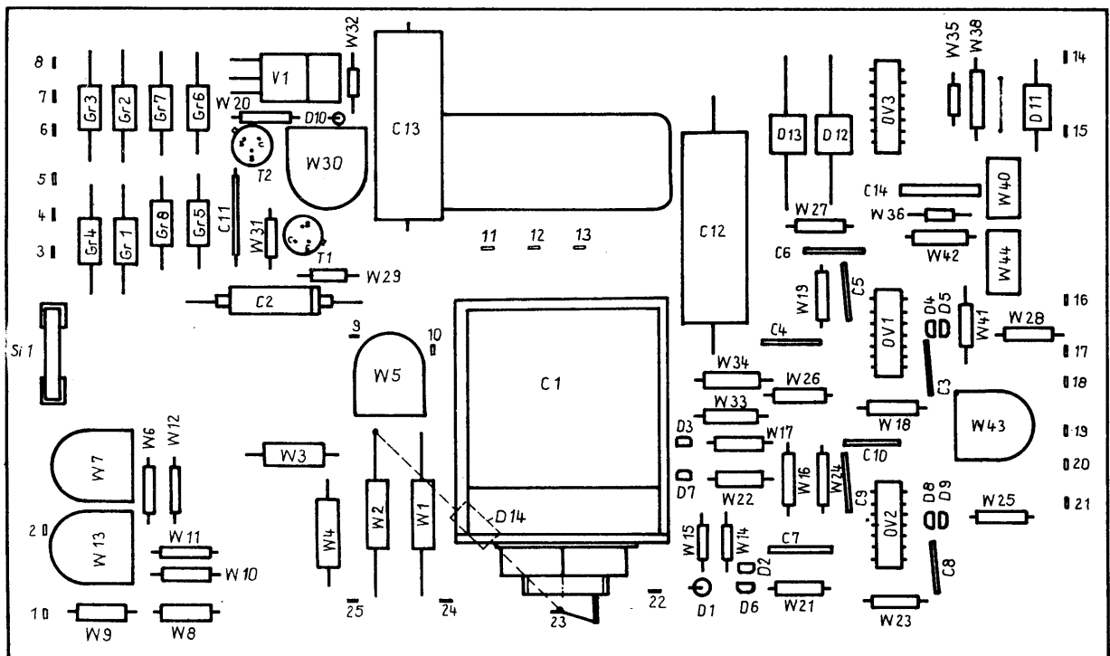
Leiterplatte
