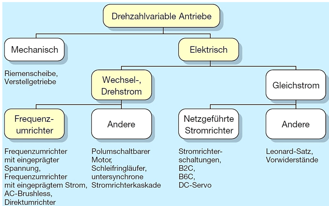
Abb. 1-1 Drehzahlvariable Antriebe 1
