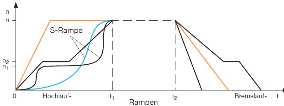
Abb. 3-2 Hochlauf- und Bremsrampen 9
