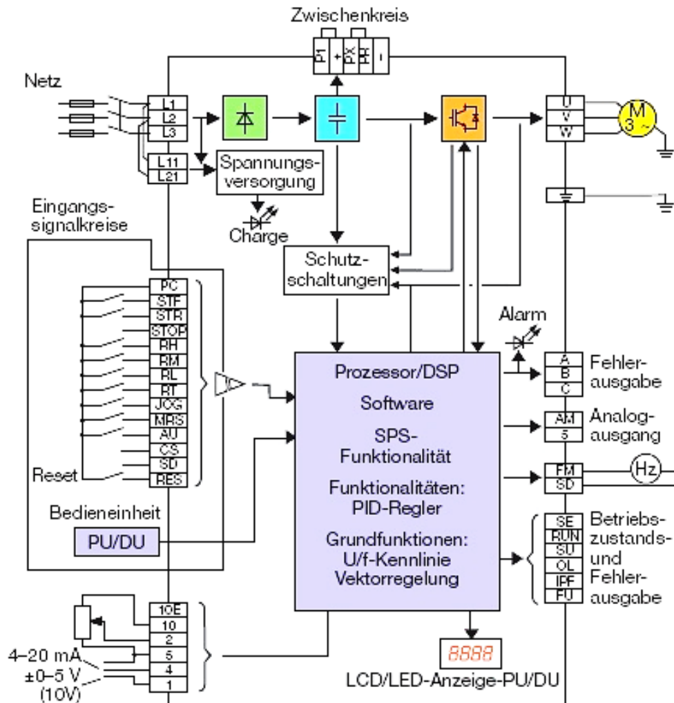
Abb. 2-1 Digitaler Frequenzumrichter 2
