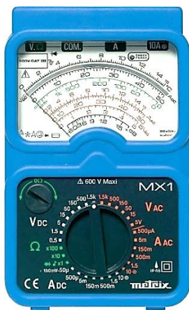
Abb. 5-4 Analog-Multimeter mit Drehspuhlmesswerk von Metex
