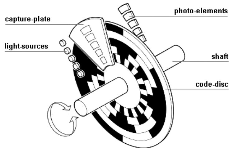
Abb. 5-11 Singleturn Encoder mit 5-Spur Gray-Code 40
