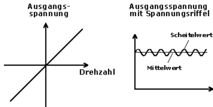
Abb. 5-3 DC-Tachospannung 34
