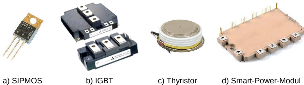
Abb. 3-7 Leistungshalbleiter
