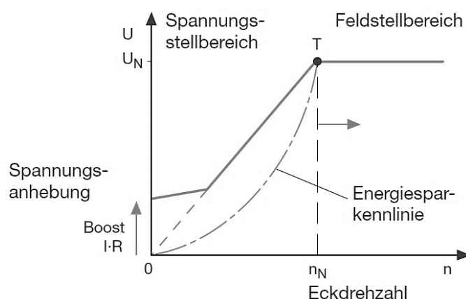
Abb. 3-1 U/f-Kennlinie 8
