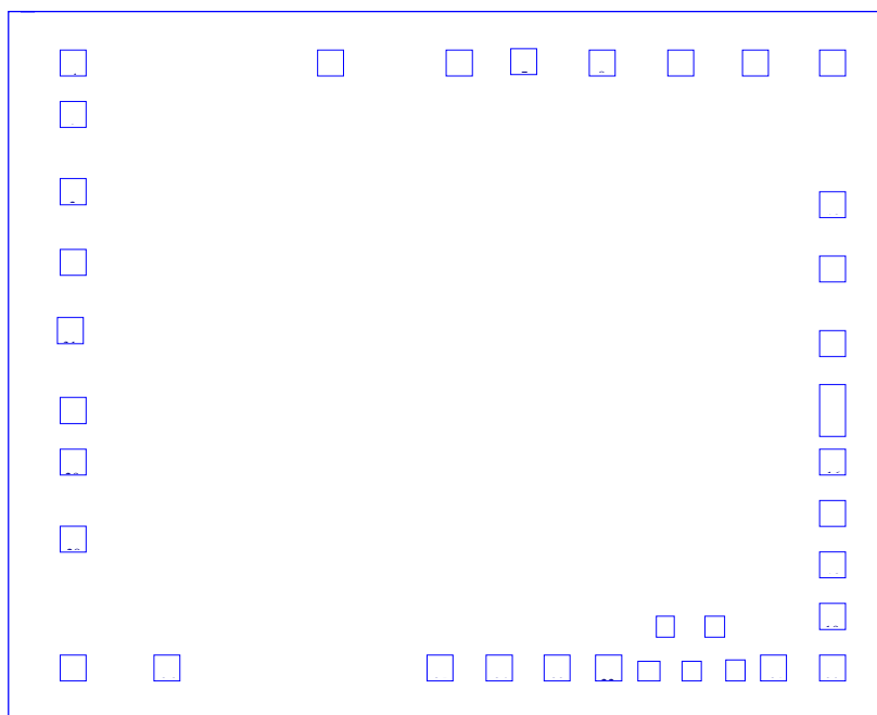
SP8560N 封装图
