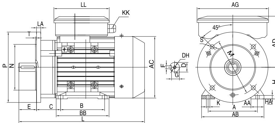
JLY/JLC/JLL IM B35
