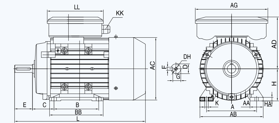
JLY/JLC/JLL IM B3
