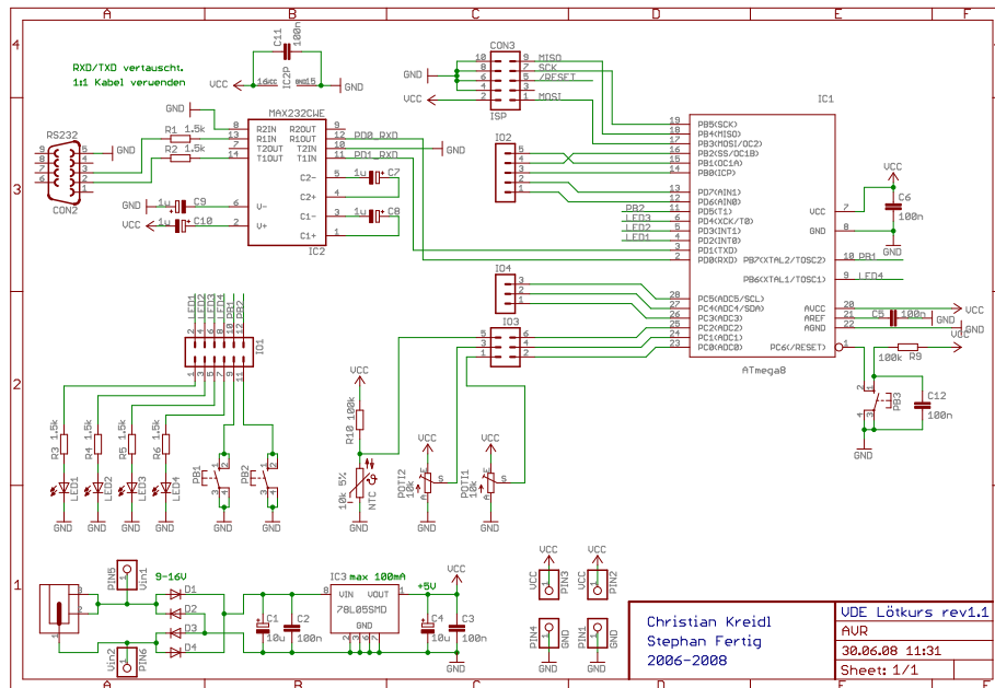
Abbildung 1: Schaltplan der \mu C-Platine
