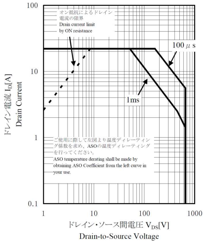
STR-X6759F MOS FET A.S.O. 曲線 curve T_a = 25^\circ\text{C} シングルプルアップ Single pluse
