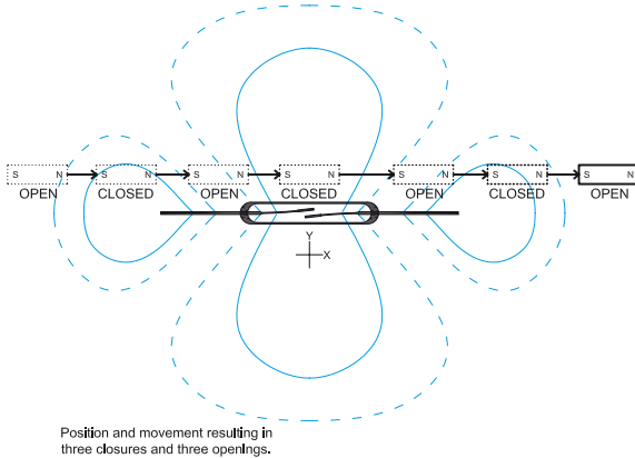
Abb. # 25 Hier werden die Punkte gezeigt, an denen der sich dem Reedschalter parallel nähernde Magnet öffnet und schließt. Der Reedschalter wird in diesem Fall drei Mal öffnen und schließt.
