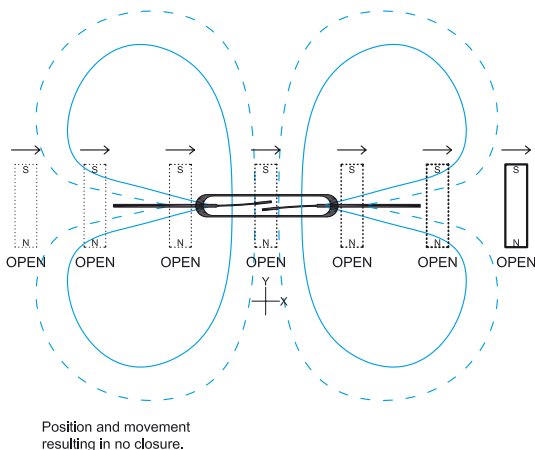
Ab. # 31 Der Magnet bewegt sich parallel zum Reedschalter auf dessen x-Achse.
