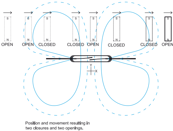
Abb. # 30 Die Schaltbereiche bei einem vertikal angeordneten Magneten mit paralleler Bewegung über den Reedschalter.
