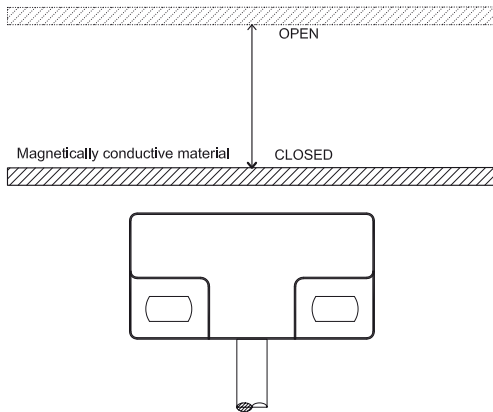
Abb. # 36 Zur Bestätigung wird kein externer Magnet benötigt. Nähert sich der Sensor einer magnetisch leitenden Fläche, so schaltet der Reedschalter. Wird diese entfernt, so öffnet er sich.
