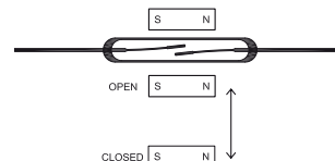
Abb. # 19 Ein Magnet bewegt sich zum Reedschalter hin oder vom Reedschalter weg.
