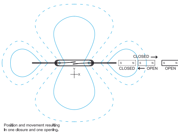
Abb. # 26 Das Schließverhalten wird beim parallelen Annähernaufgezeigt.
