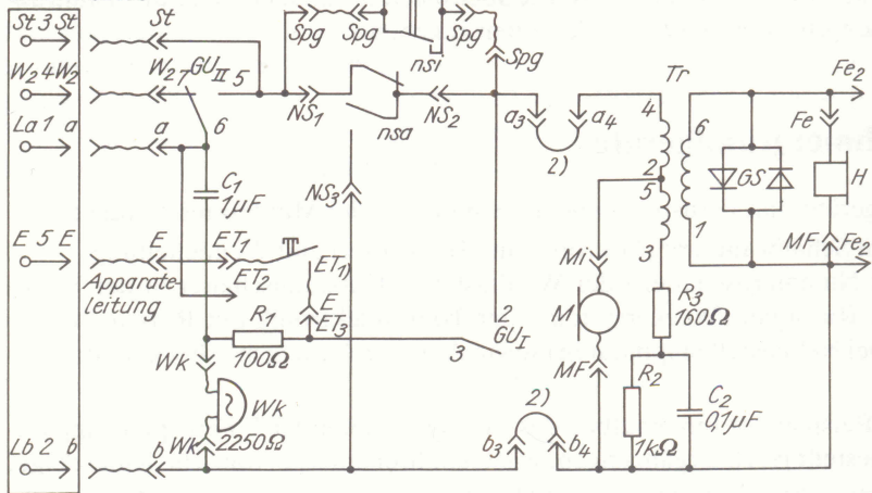
Bild 9.2 Fernsprechapparat Variant, Apparateschaltung
