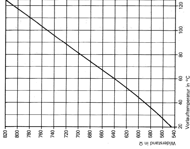
Vorlauftempersensor, Best.-Nr. 7270 144
