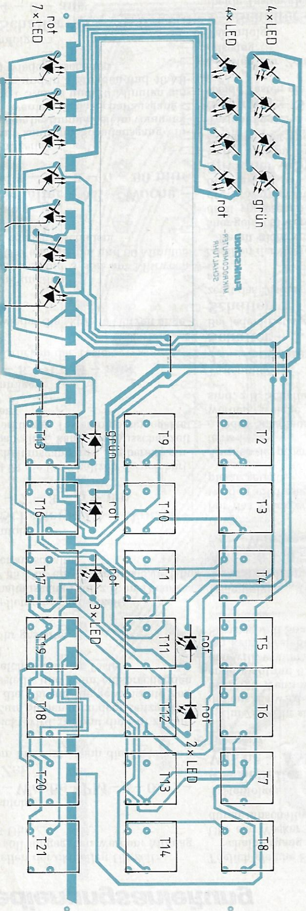
Bild 9. Bestückungsplan für die Frontplatte in Bild 8. Die erforderlichen Brücken sind auf der Leiterbahnseite mit isoliertem Draht herzustellen
