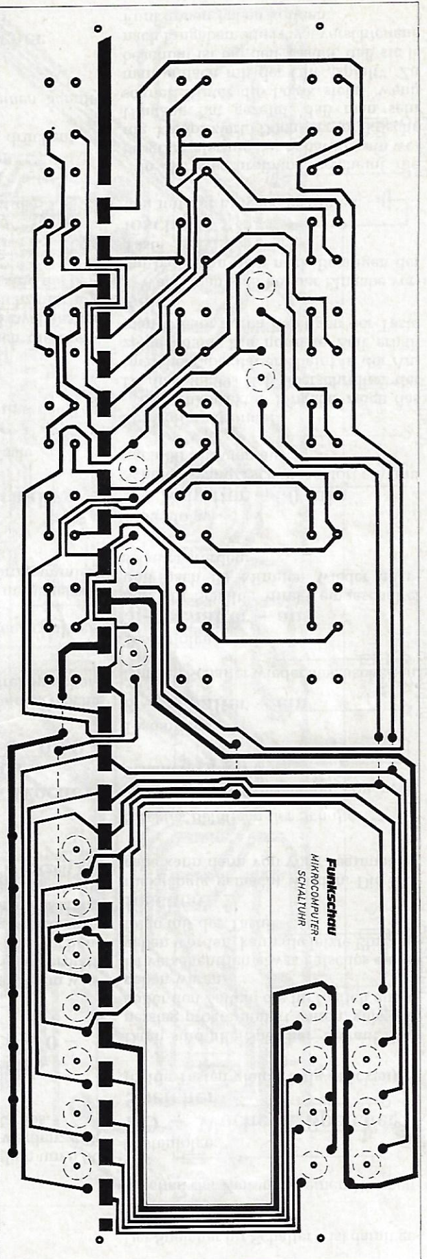
Bild 8. Die Platine für das Tastenfeld der Mikrocomputer-Schaltuhr ist gleichzeitig die Frontplatte für das Gehäuse
