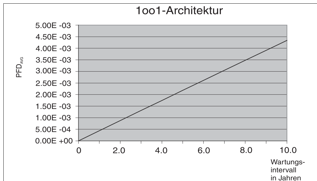
Abb. 4: "Mittlere Wahrscheinlichkeit gefährbringender Ausfälle des sicherheitsbezogenem Systems auf Anforderung" ( PFD_{AVG} ) in Abhängigkeit vom gewählten Wartungsintervall
