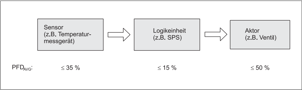
Abb. 1: Übliche Aufteilung der "mittleren Wahrscheinlichkeit gefährbringender Ausfälle einer Sicherheitsfunktion im Anforderungsfall" ( PFD_{AVG} ) auf die Teilsysteme
