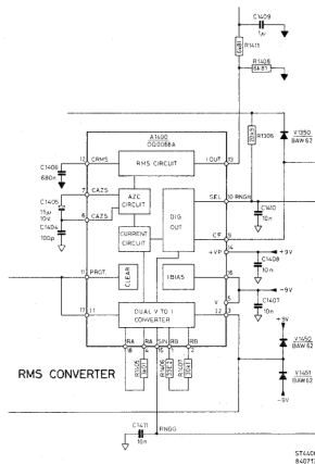
Fig. 2.9. RMS converter
