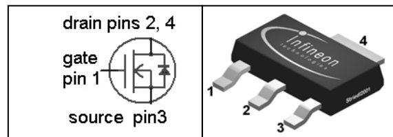
SOT-223
