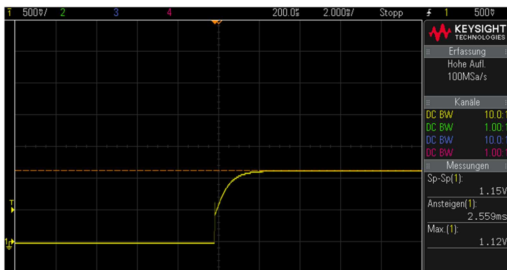
Abbildung 3: Turn on – CC-Mode 40mA
