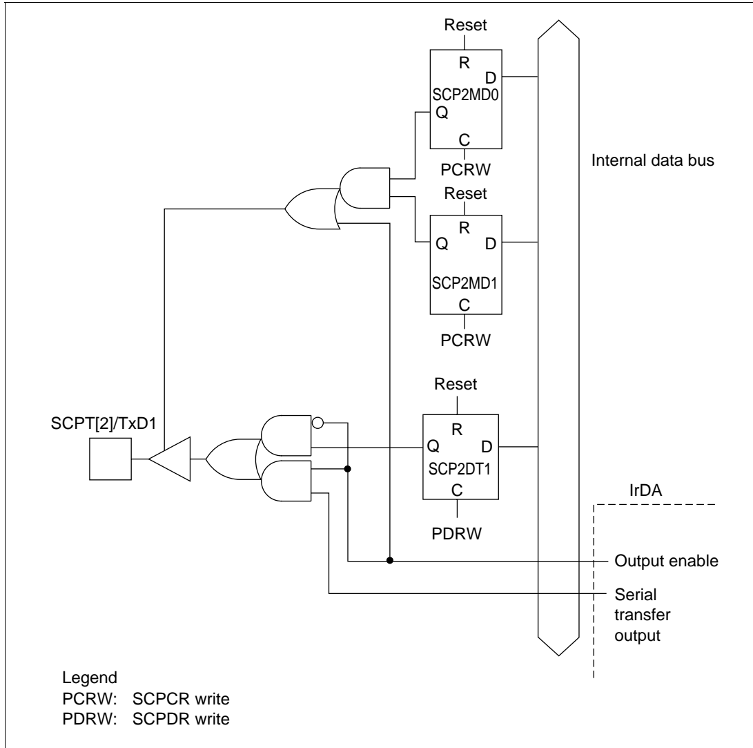
Figure 17.3 SCPT[2]/TxD1 Pin
