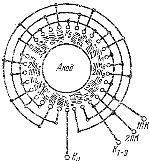
Схема расположения электродов в двухимпульсных декатронах
