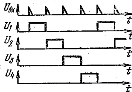
Диаграмма управляющих импульсов напряжений прибора ИН-26
