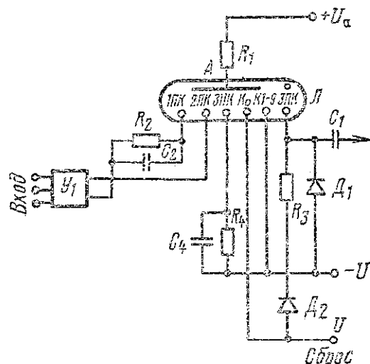
Типовая схема включения одноимпульсных декактронов с симметричными катодами:
