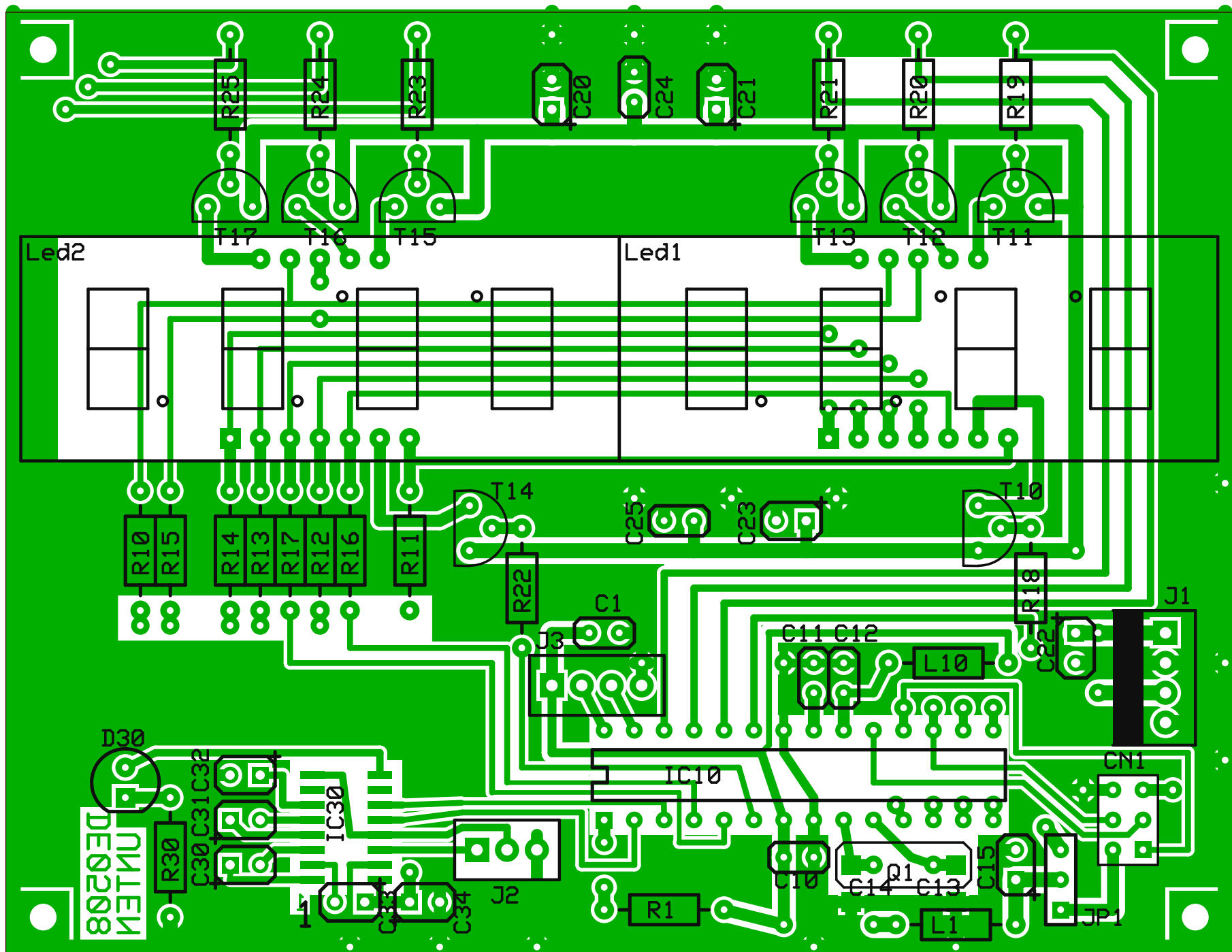
FR4, 2-seitig, LxB 104,14mm x 80 mm
