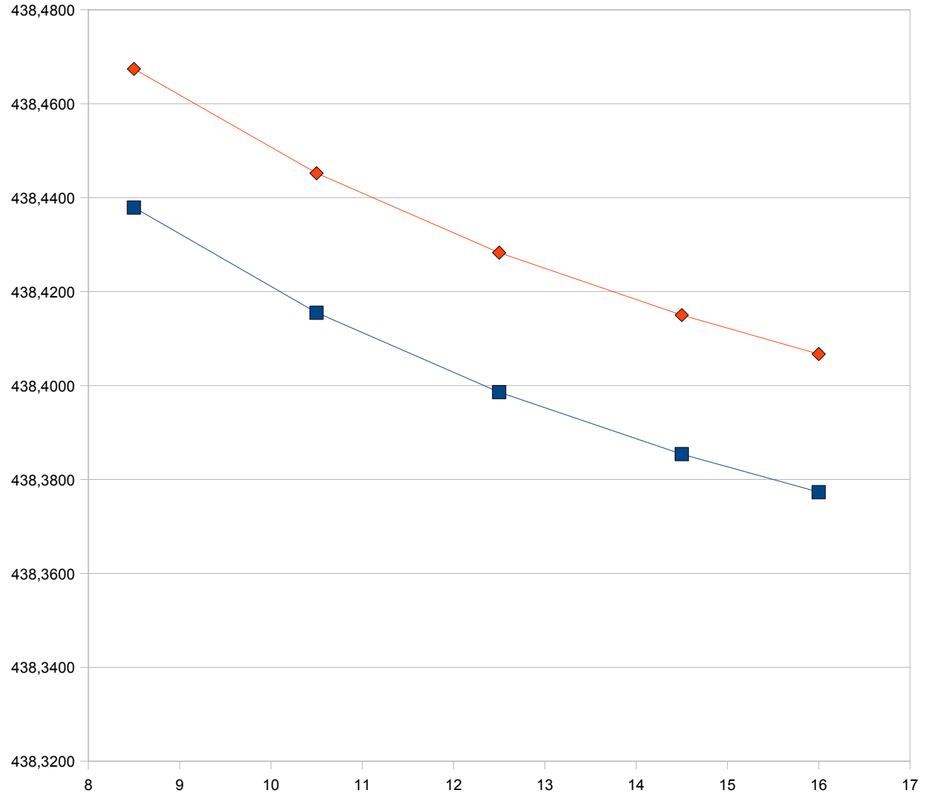
Feinverstimmung der Frequenz im RFM12 durch Änderung der Oszillatorkapazität, oben mp=1, unten =0
