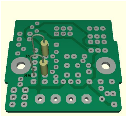
Abbildung 15: R5, R6 (1,5kΩ)
