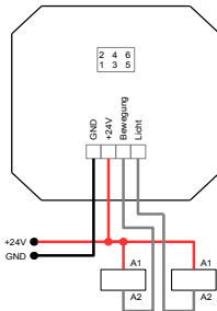
Abbildung 3: low side Ausgangssbeschriftung bei gleicher Lastspannung
