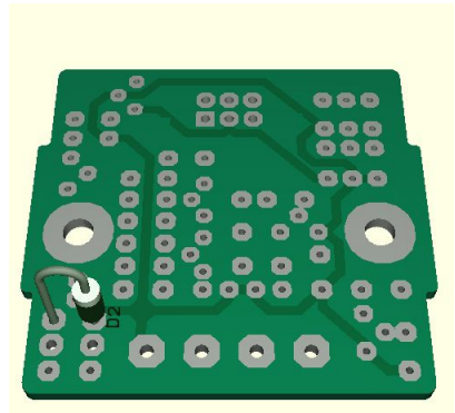
Abbildung 6: D2 (P4KE33A)
