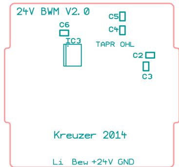
Abbildung 29: Bestückungsdruck unten
