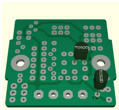
Abbildung 11: T3, T4 (BC547B)
