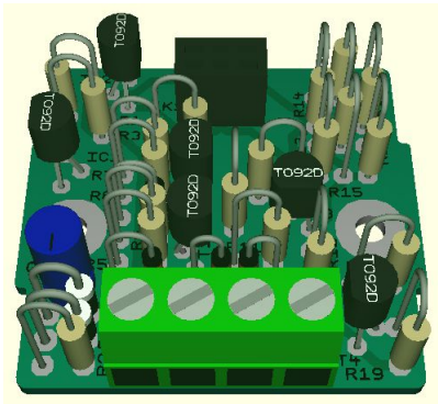
Abbildung 23: komplett Bestückt
