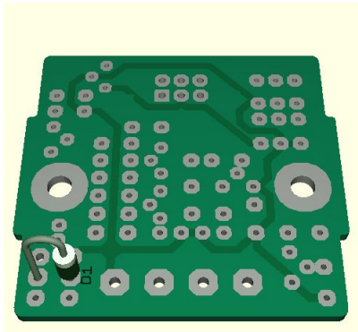
Abbildung 5: D1 (1N4007)
