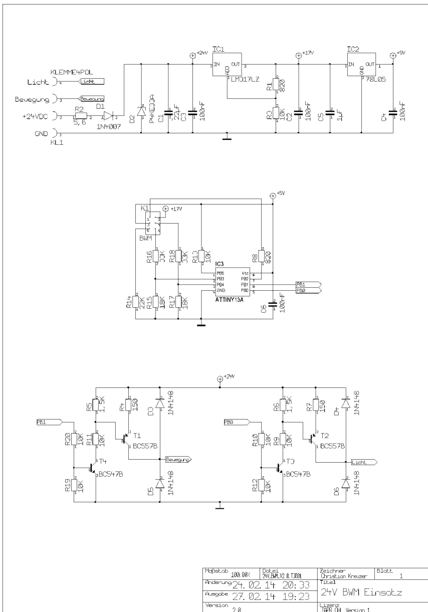
Abbildung 27: Schaltplan
