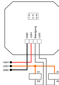
Abbildung 4: low side Ausgangssbeschriftung bei geringerer Lastspannung
