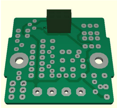
Abbildung 21: K1 (2x3)
