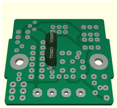
Abbildung 10: T1, T2 (BC557B)
