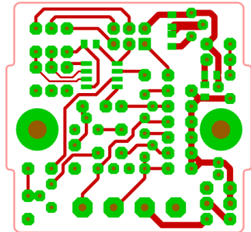
Abbildung 31: Kupfer, Lötstopp unten
