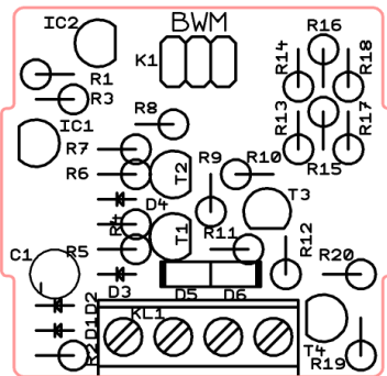
Abbildung 28: Bestückungsdruck oben
