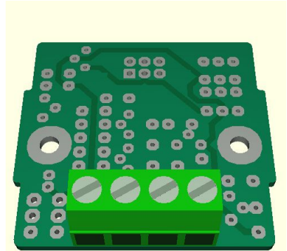
Abbildung 22: KL1 (2x5,08)
