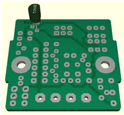
Abbildung 9: IC2 (78L05)
