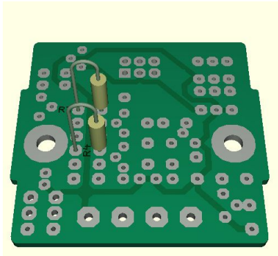
Abbildung 13: R4, R7 (150Ω)
