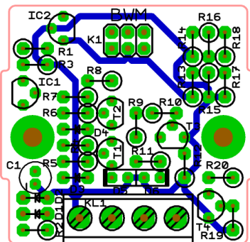
Abbildung 32: Layout oben
