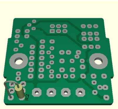
Abbildung 12: R2 (5,6Ω)
