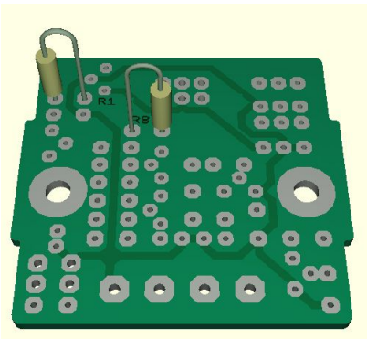
Abbildung 14: R1, R8 (820Ω)
