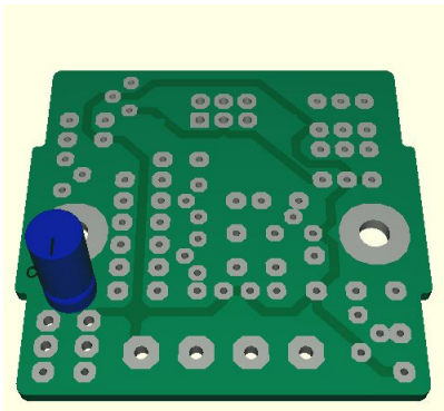
Abbildung 20: C1 (22 \mu F)
