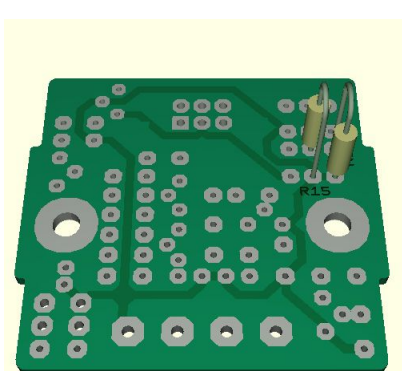
Abbildung 17: R15, R17 (18kΩ)
