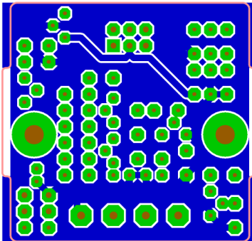
Abbildung 30: Kupfer, Lötstopp oben
